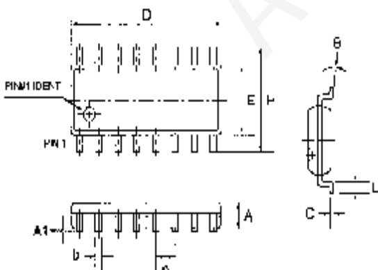
贴片封装外观尺寸 (SOP 16L)
